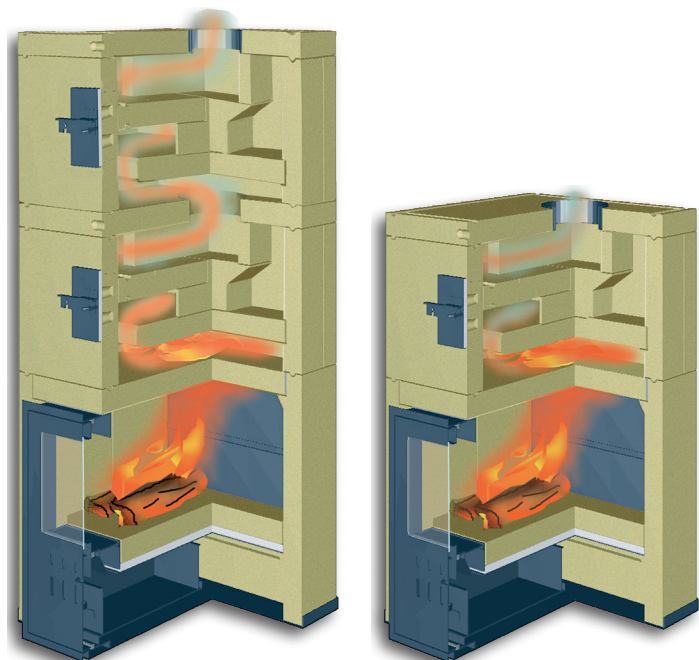
Cubolino plus / Cubolino Funktionsschema
