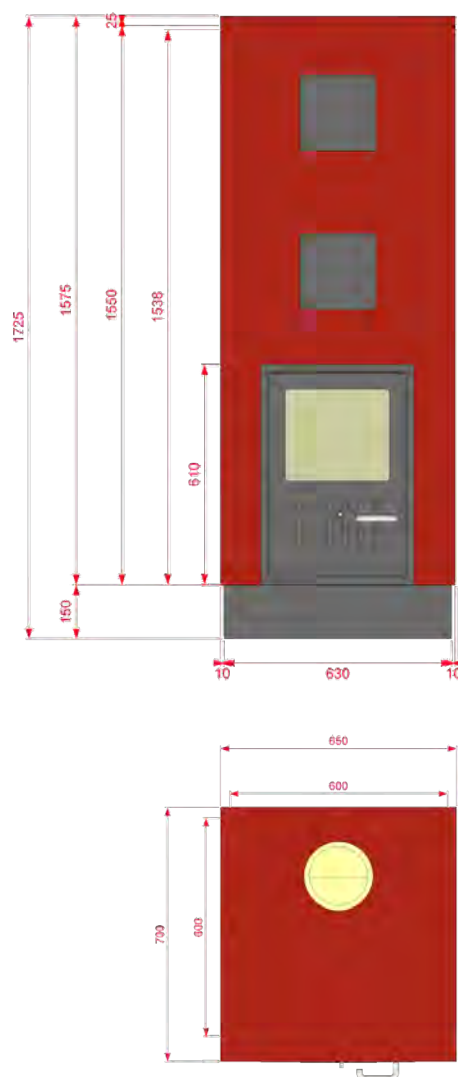
Ansicht Front mit Abmessungen Cubolino Comfort
